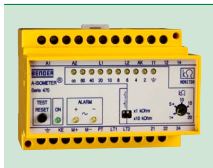
ISOMETER® IR470LY
