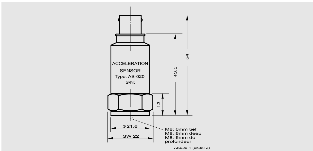
Abb. 1 Beschleunigungs-Sensor AS - 020
