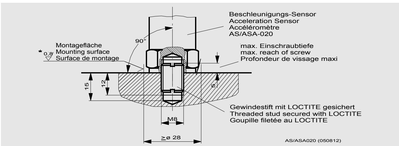
Abb. 3 Montage
